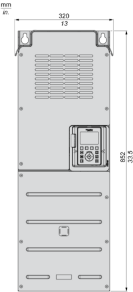
Variadores sin cubierta superior IP21 Vistas lateral derecha y frontal
